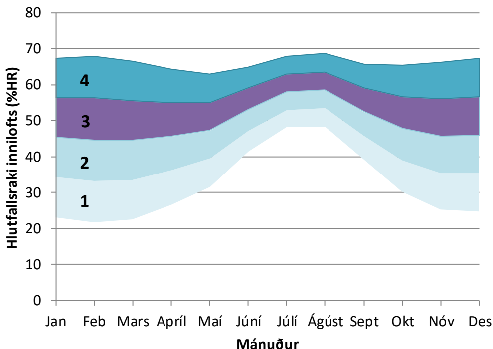
Mynd 3. Reiknaður hlutfallsraki lofts innanhúss í Reykjavík fyrir mismunandi rakabætingu (0-8 g/m 3 ) og innihita 20°C. Útiaðstæður eru meðaltal áráanna 1996-2004.
