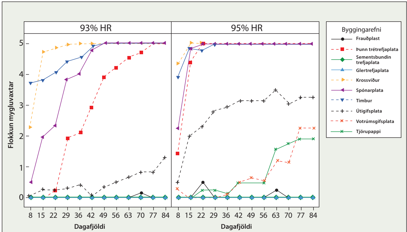
Mynd 5. Niðurstöður rannsókna á 10 algengum byggingarefnum í Svíþjóð.
