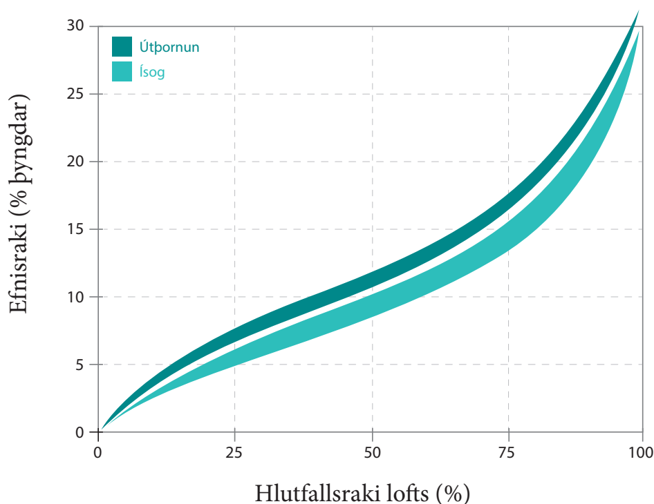
Mynd 6. Dæmigerður jafnvægisraki barriðar.
