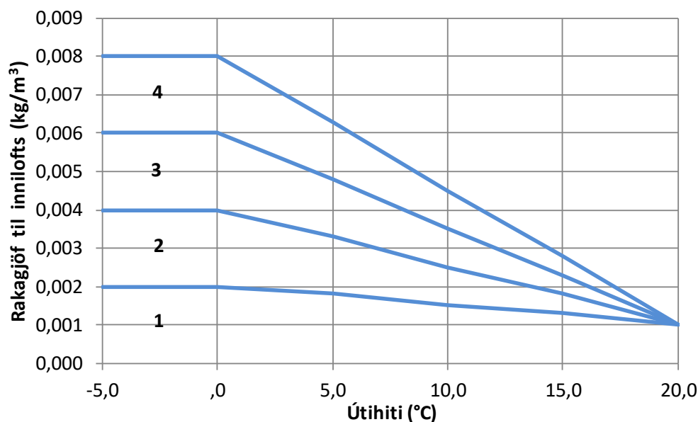
Mynd 2. Reiknisleg rakabæting í inniloft; (0-8 g/m 3 loftskiptum) (Heimild: ÍST EN ISO 13788:2012).
