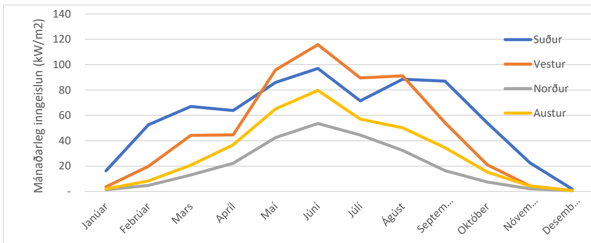
Mynd 11: Reiknuð framleiðsla mánaða m.v. 1 kW uppsett afl; áhrif a) halla á panel snúandi í suður og b) stefnu sólarpanels með 90° halla við 64°N fyrir viðmiðunarárið september 2018 til ágúst 2019.
