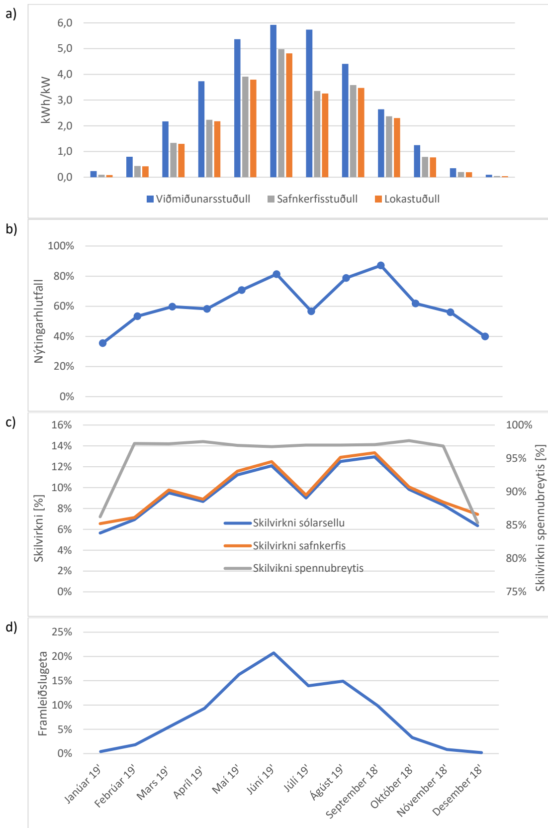
Mynd 13: Frammistaða sólarorkukerfis IKEA á fyrstu 12 rekstrarmánuðum.
