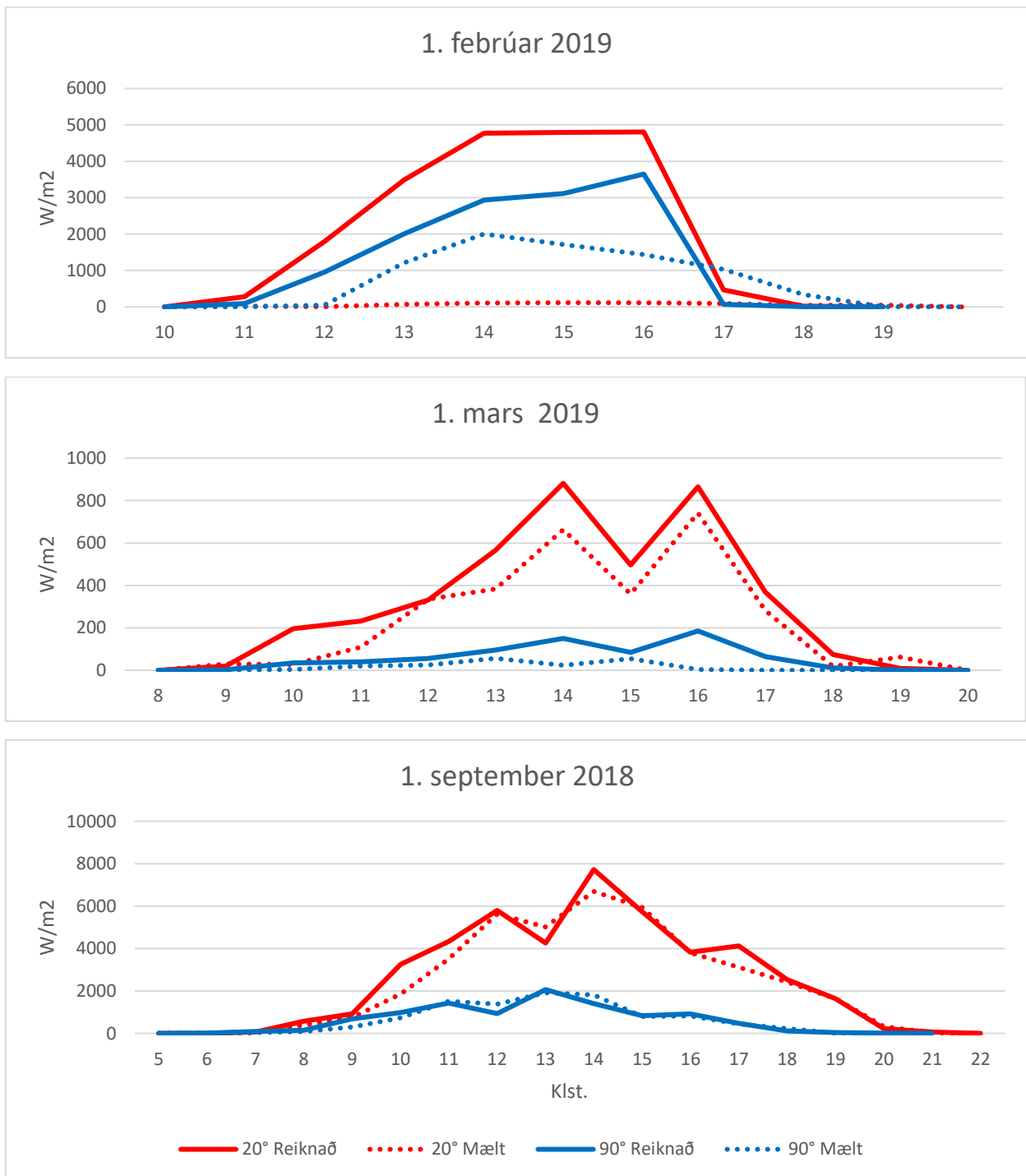
Mynd 10: Samanburður á mældri (heil lína) og reiknaðri (brotalína) sólarinngeislun á þremur dögum.
