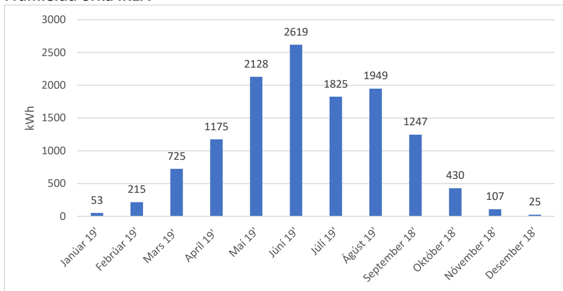
Mynd 12: Framleidd orka frá safnkerfinu hjá IKEA
