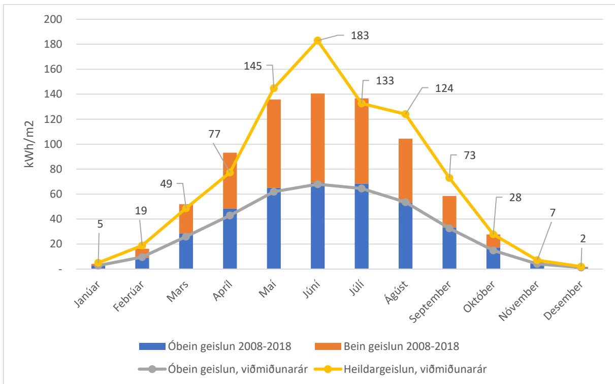
Mynd 4: Mánaðarleg meðalgeislun á láréttan flöt í Reykjavík á árunum 2008-2018 ásamt viðmiðunarári skipt í beina og óbeina geislun. Gögn: Veðurstofa Íslands (2019)
