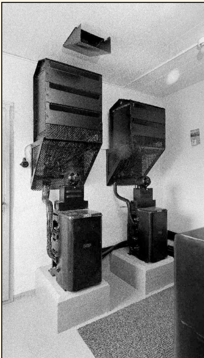
Hraðastýribúnaður fyrir stöðina. (Ljósmyndari Guðmundur Ingólfsson - Árbæjarsafn)
