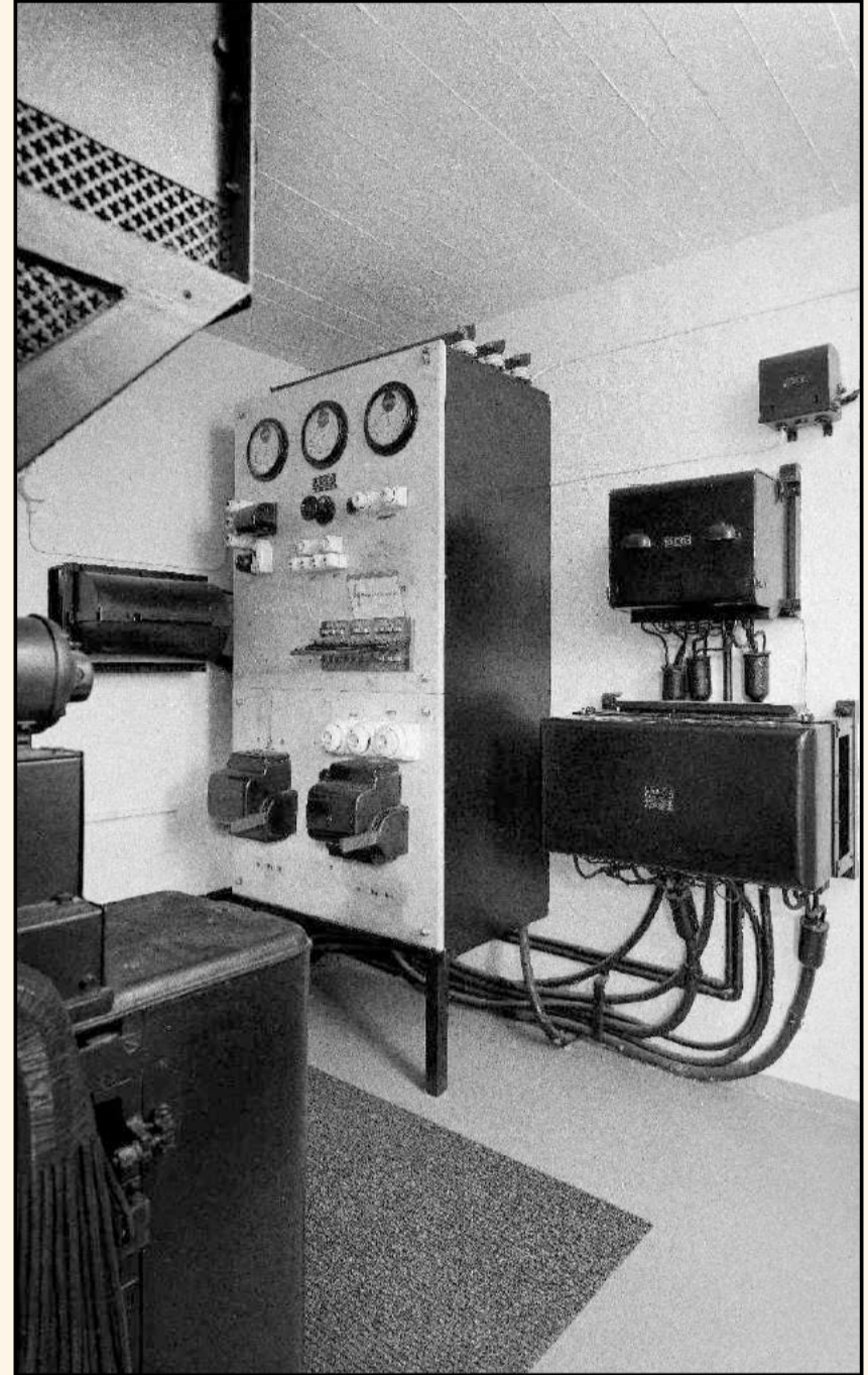
Rafmagnstafla fyrir stöðina. (Ljósmyndari Guðmundur Ingólfsson - Árbæjarsafn)
