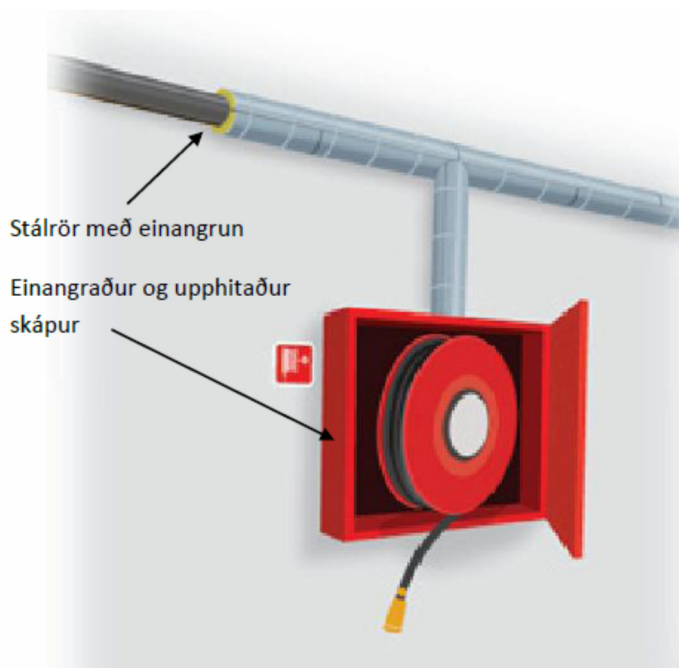
Mynd 4 Stálrör með hitaþræði og einangrun að einangruðum og upphituðum skáp fyrir slöngukefli þar sem frosthætta er. Mynd af www.rockwool.dk
