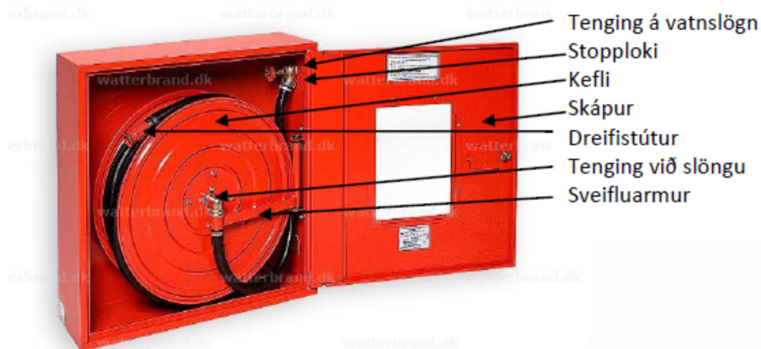
Mynd 2 Dæmigert slöngukefli í skáp. Einnig eru til slöngukefli sem eru fest innan á skáphurðina. Mynd af www.watterbrand.dk
